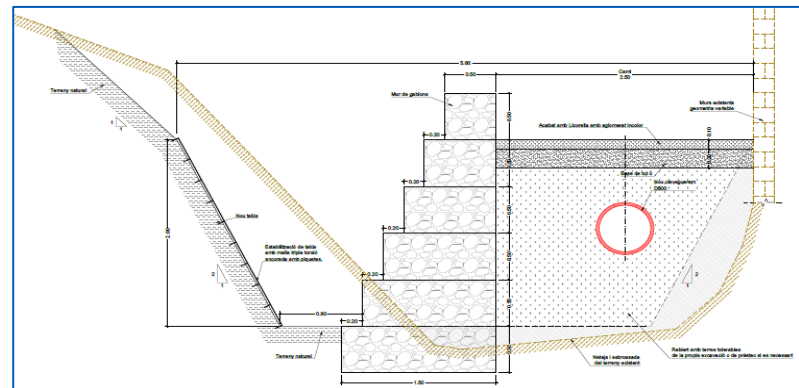
Secció tipus adequació Torrent dels Arcs
